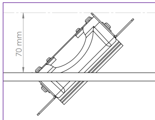
Fig. 2: Gipsarmatuur schuin door het gat steken. Minimale montagehoogte 70 mm
