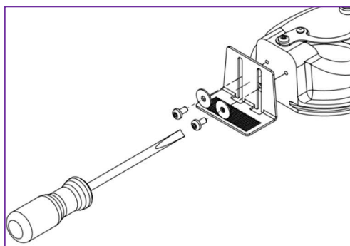
Fig. 3: Montagehoeken bevestigen op de juiste hoogte.
