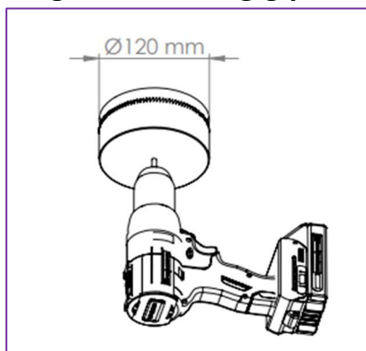
Fig. 1: Gat zagen \varnothing 120 mm
