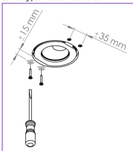
Fig. 4: Vast schroeven gipsarmatuur in het plafond
