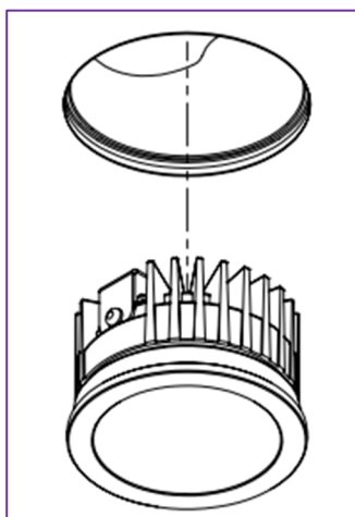
Fig. 8: Plaats led-spot of aanwezigheidsmelder in het gipsarmatuur.
